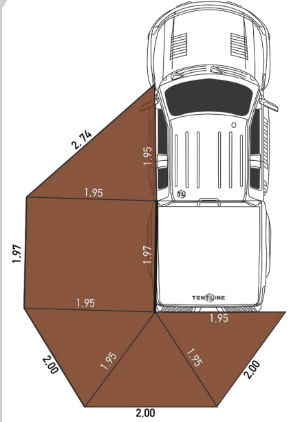
6 BRAZOS 270°
